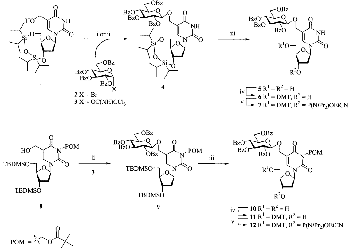
Scheme 1. Reagents and conditions: (i) for 2 : HgBr 2 , Hg(CN) 2 , ACN, 3 h, 50%. (ii) for 3 : cat. TMSOTf, DCE, 1.5 h, 4 : 47%, 9 : 96%. (iii) Et 3 N·3HF, pyridine, 16 h, 5 : 90%, 10 : 91%. (iv) DMTCl, pyridine, 3 h, 6 : 71%, 11 : 75%. (v) ClP(NiPr 2 )OEtCN, DIPEA, DCM, 1 h, 7 : 69%, 12 : 91%
